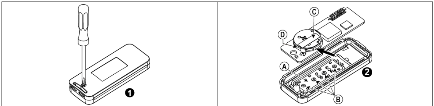
Reemplazo de la batería Sostituzione della batteria Figura 2
